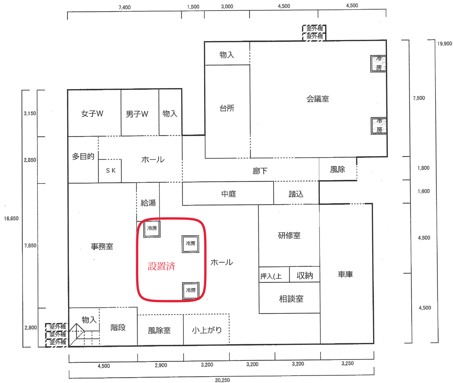
森町交流支援センター平面図 2箇所
