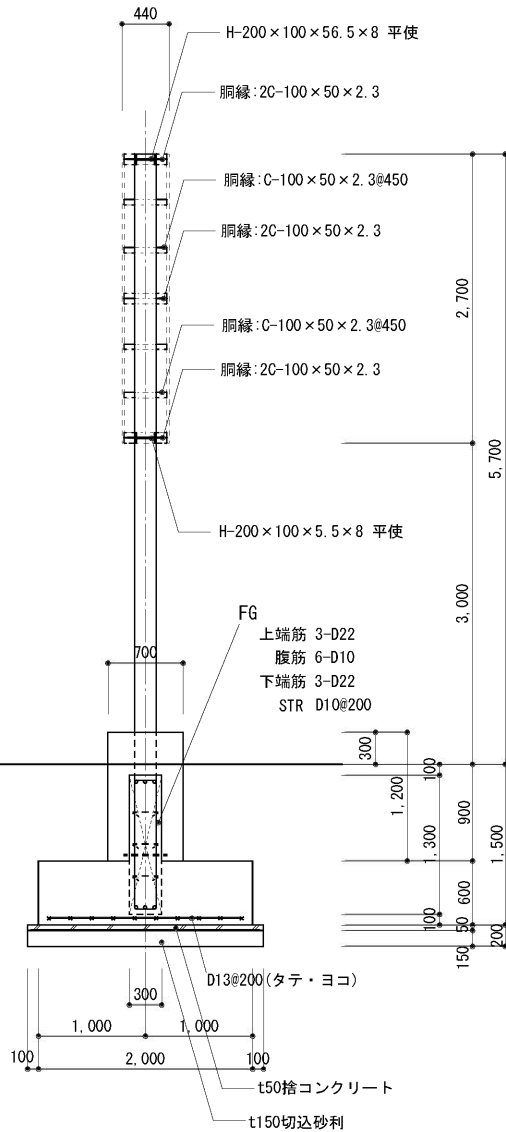
断面図・構造詳細 S=1:50
