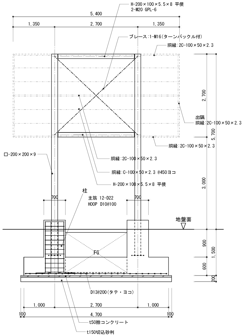
断面・構造詳細図 S=1:50
