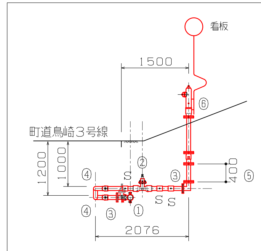
側面図
