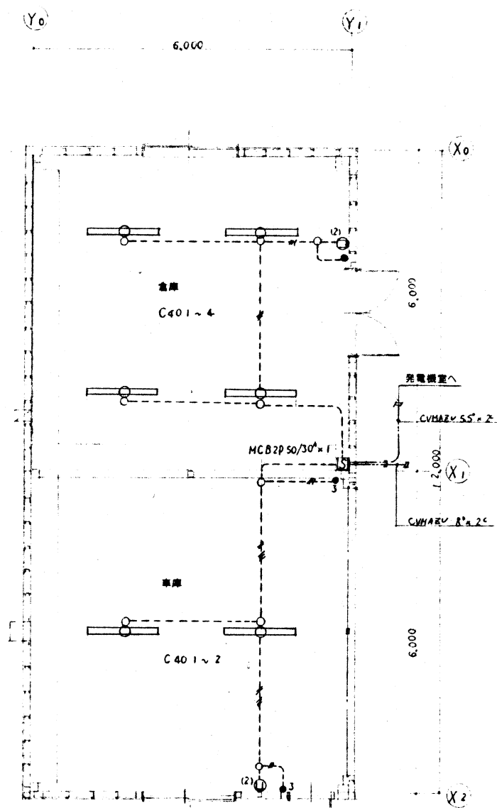
平面図 S=1:50
