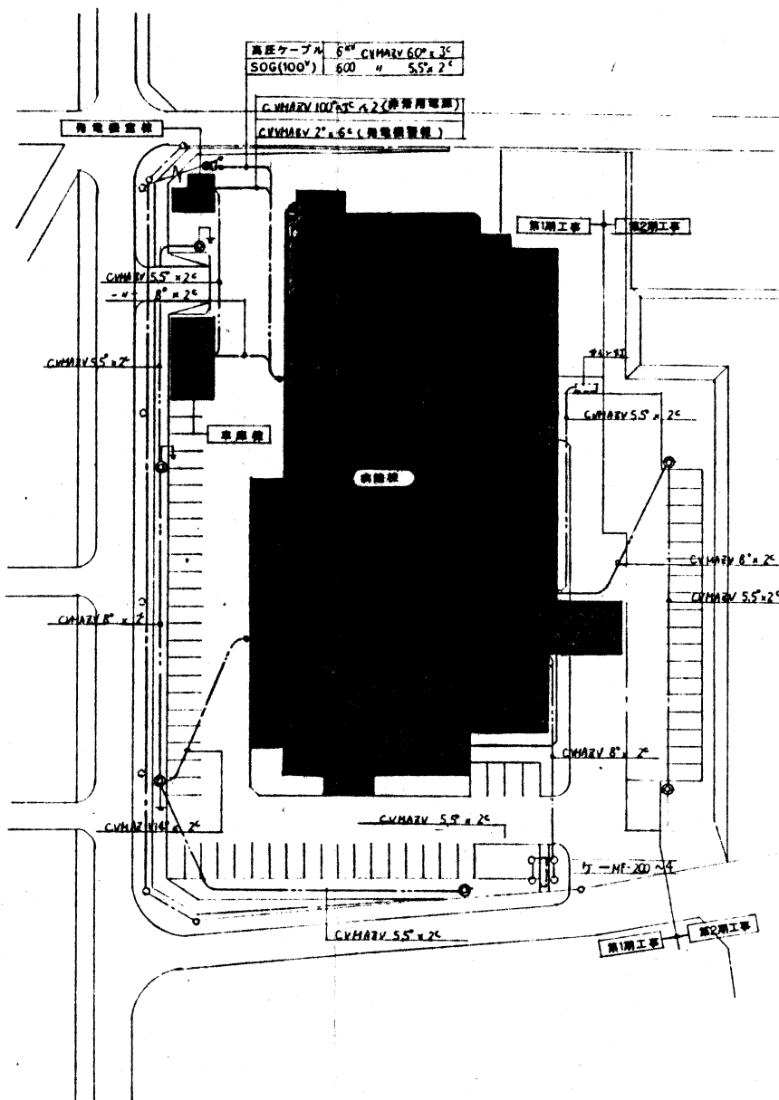
配置図 S=1:500
