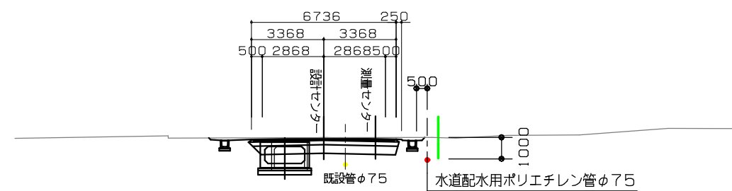
φ75横断図 S=1/100
