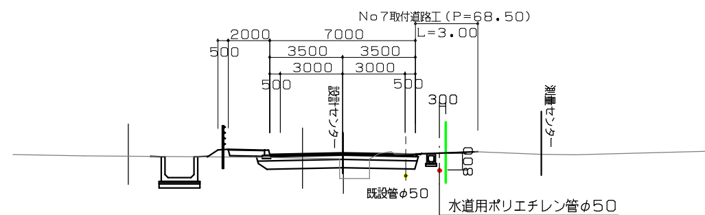
φ50横断図 S=1/100
