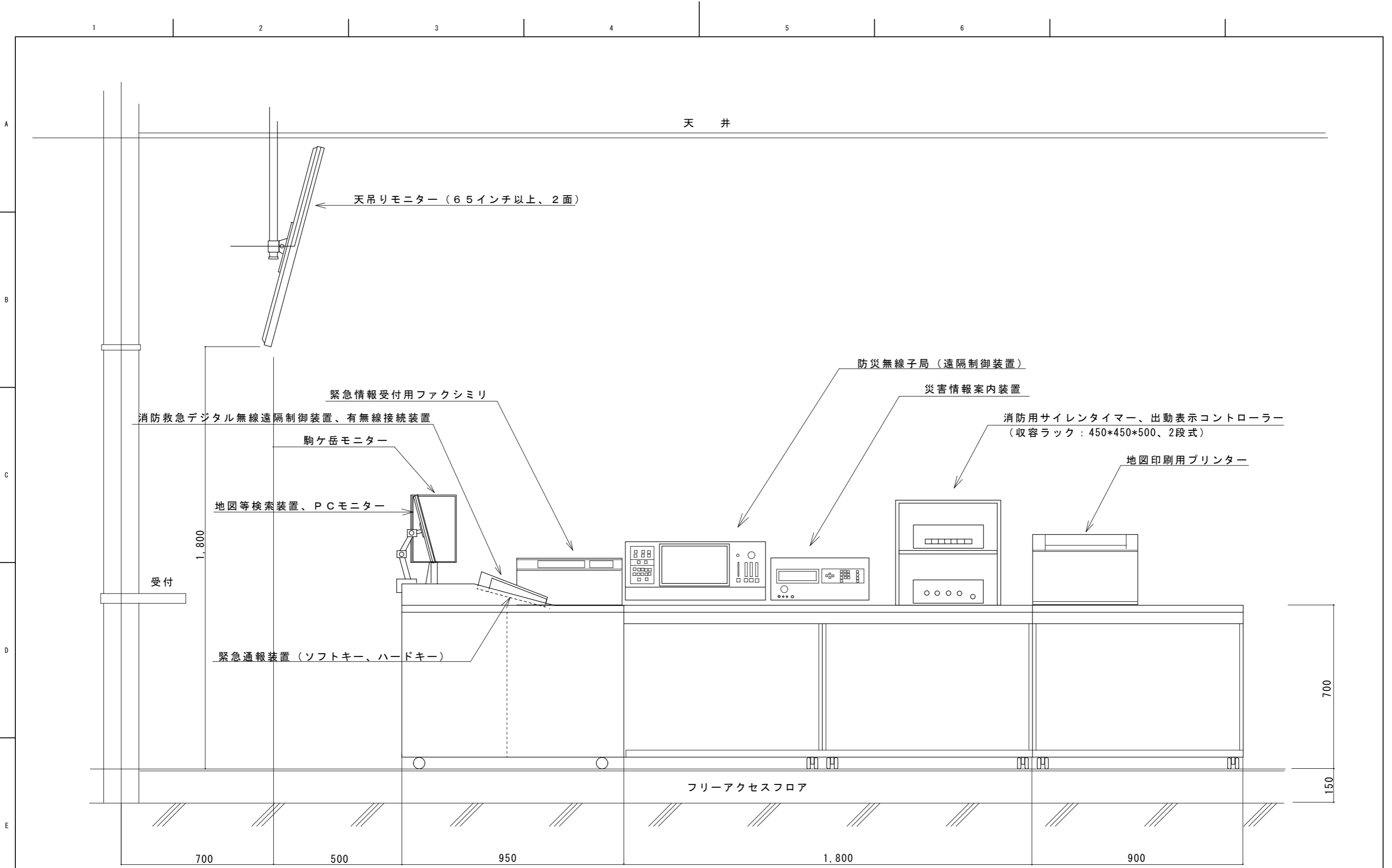
矢視 A
