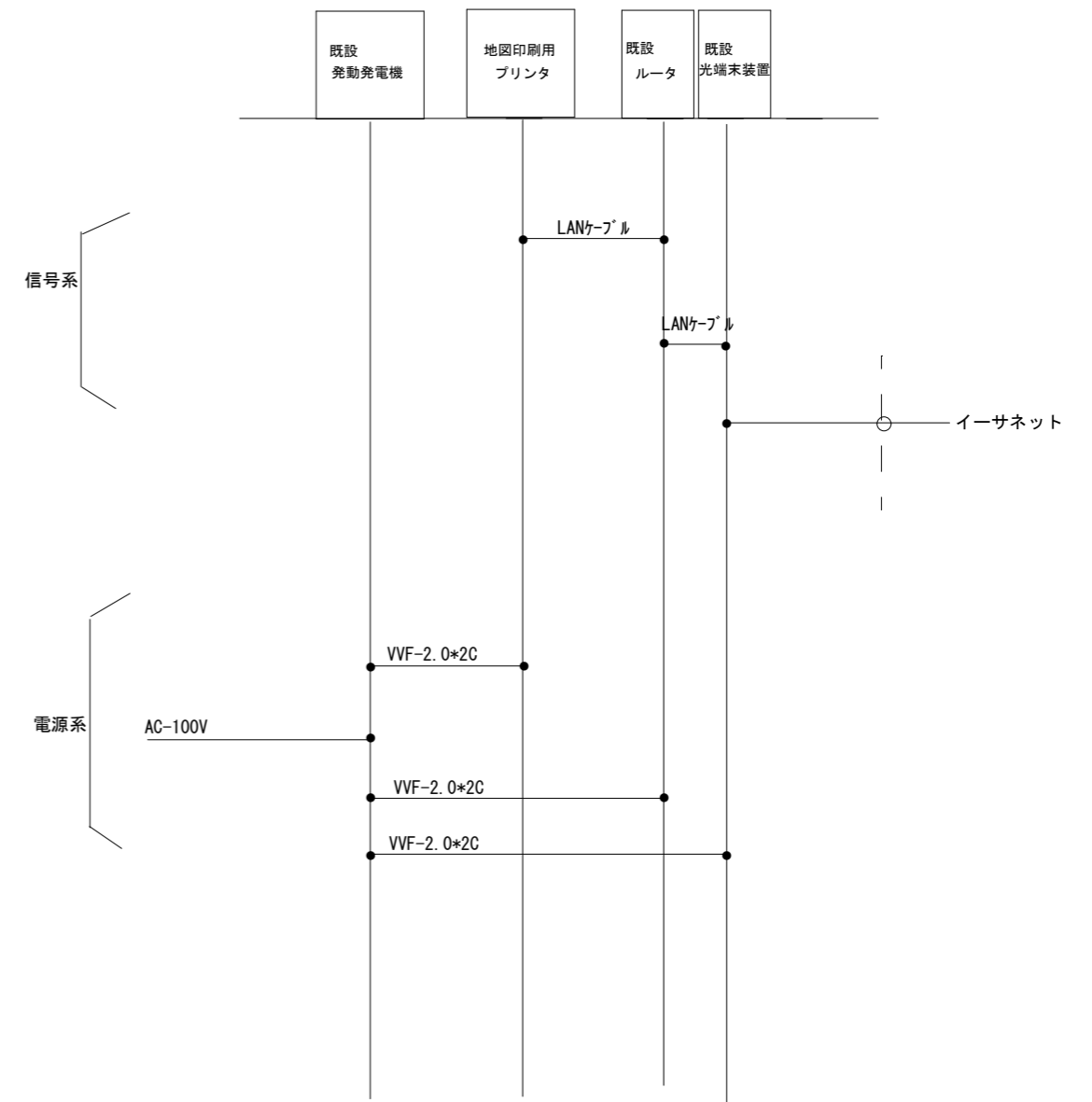
信号・電源系統図
