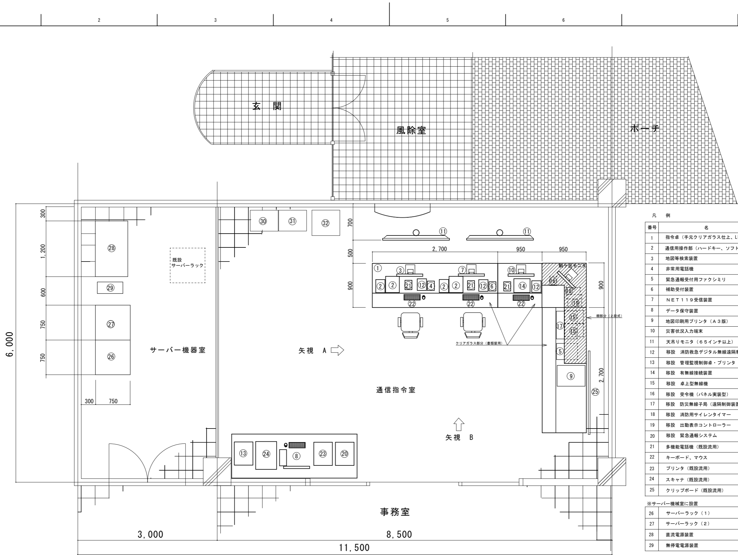
通信指令室 平面図 (1/50)
