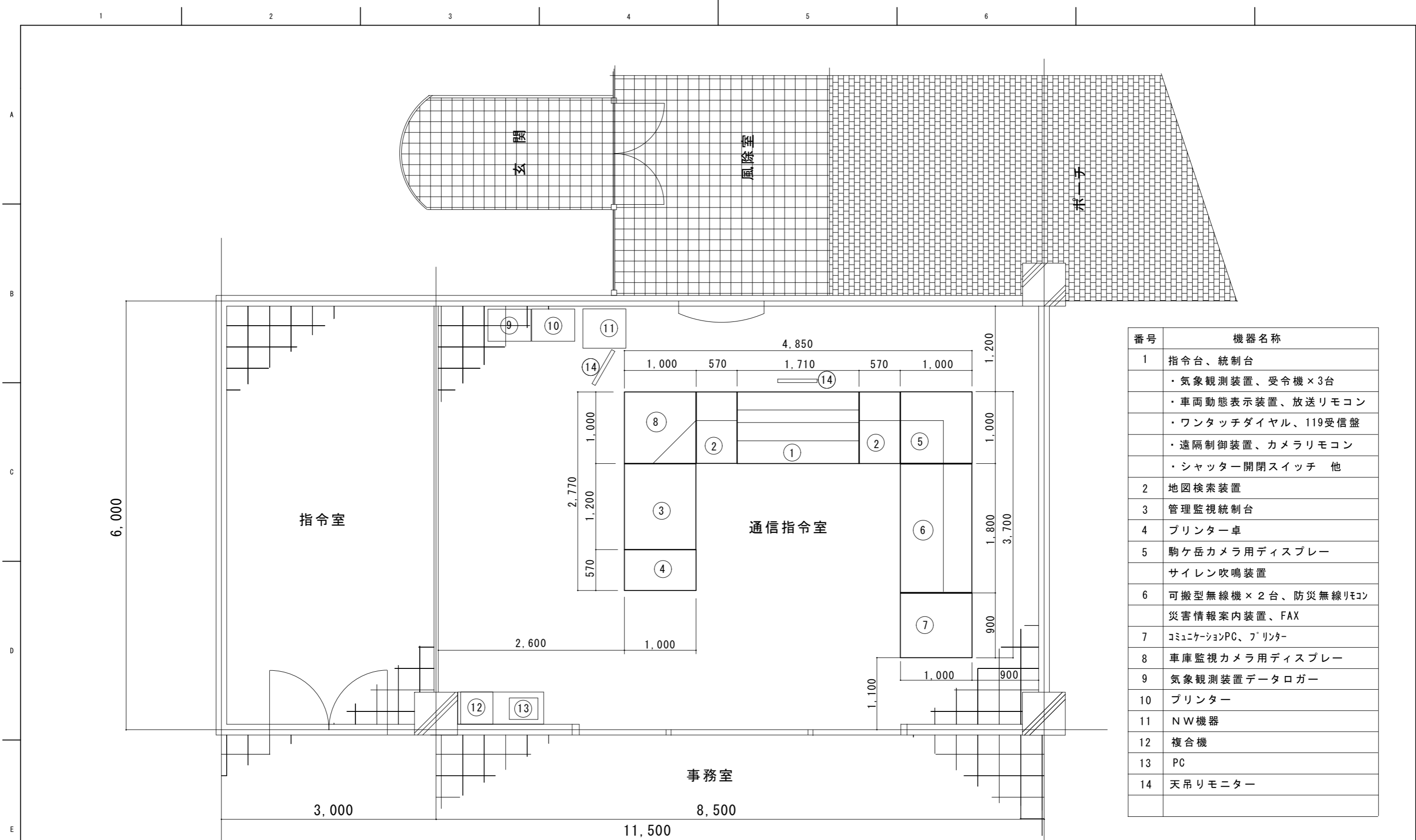
通信指令室 平面図 (1/50)
